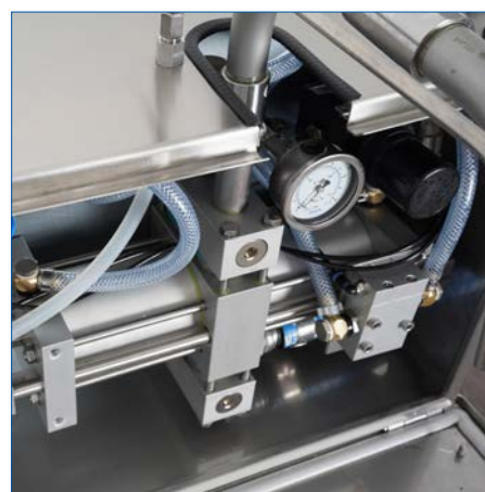
Harzpumpe und Druckregleinheit
