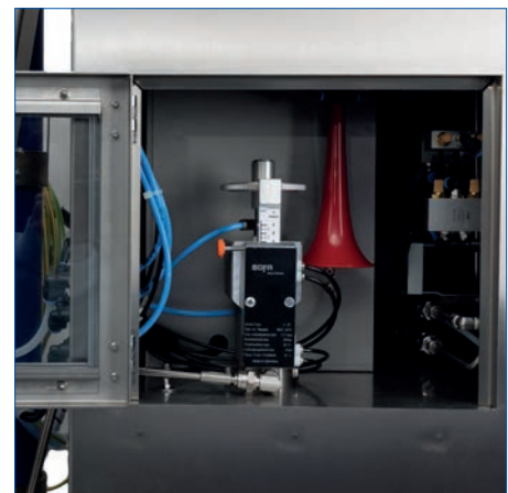
Härterpumpe
