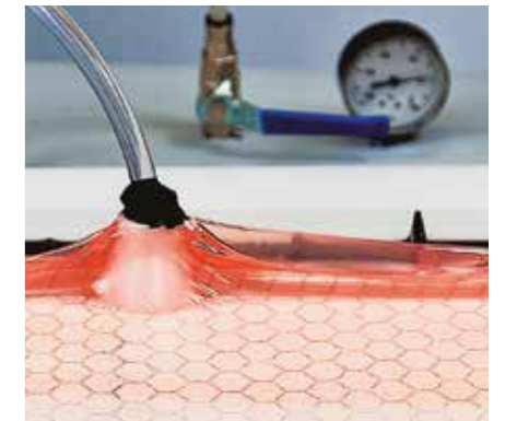
Infusionsaufbau
